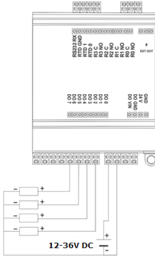
Şekil 11 RTU300 Dijital Çıkış Bağlantı Şeması
